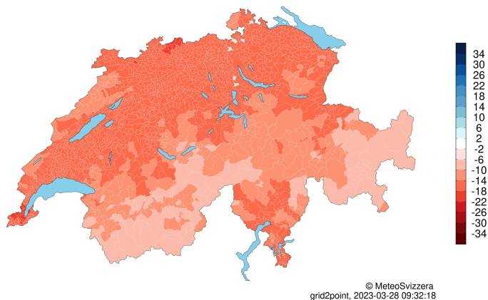
Deviazione dei gradi giorno di riscaldamento risp. al 1991-2020 [%] Periodo 1.10.2022 - 27.3.2023
