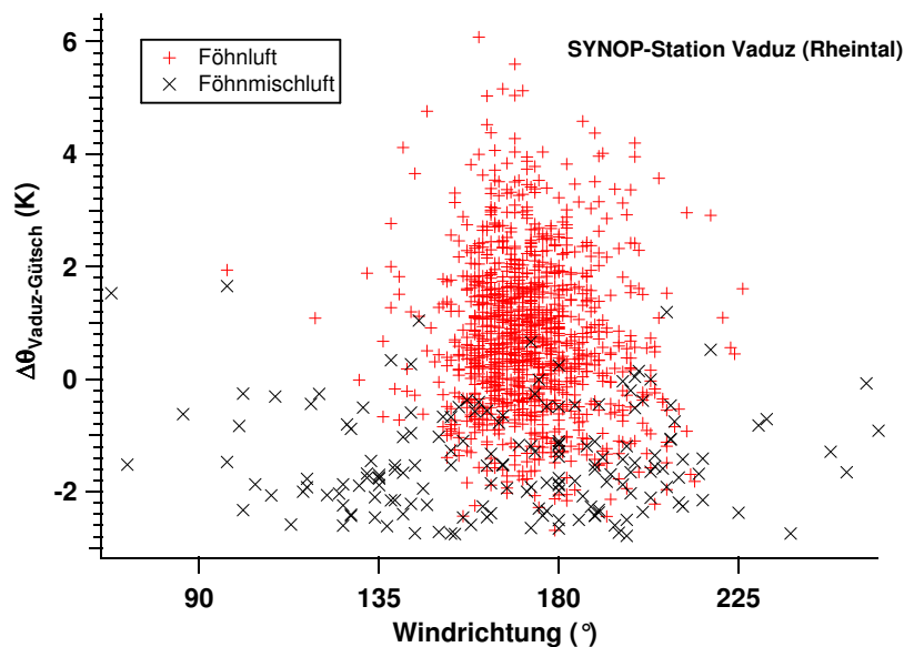
Abbildung 3: Föhnluft und Föhnmischluf in Vaduz von 1991 – 2000. Es sind jeweils nur die Zehnminutenwerte alle 3 Stunden angegeben, d.h. um 0000 UTC, 0300 UTC, 0600 UTC usw. Die Föhnmischluf unterscheidet sich von der Föhnluft in Vaduz durch niedrigere potentielle Temperaturen bezüglich Gütsch und durch eine grössere Streuung der Windrichtung bezüglich der Hauptwindrichtung.
