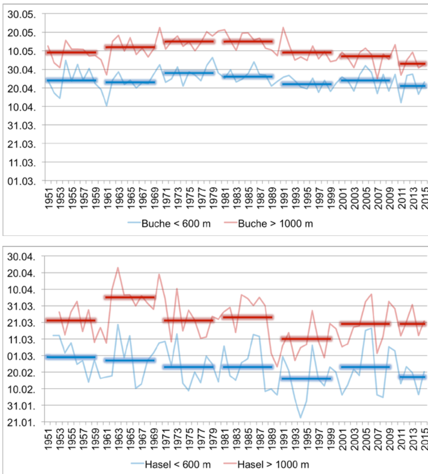
Abbildung 1: Entwicklung der Blattentfaltung bei der Buche (oben) und der Blüte bei der Hasel (unten) zwischen 1951 und 2015 für Standorte der tiefen Lagen (< 600 m ü. M) und der hohen Lagen (> 1000 m ü. M). Dargestellt sind die einzelnen Jahreswerte sowie die Mittel der Dekaden (10-Jahres-Perioden). Quelle: Bundesamt für Meteorologie MeteoSchweiz und PhaenoNet 2016
